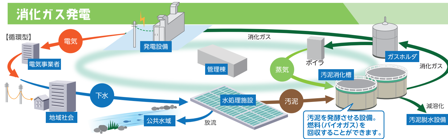
【マルツ越前家久浄化センター消化ガス発電所フロー図】
